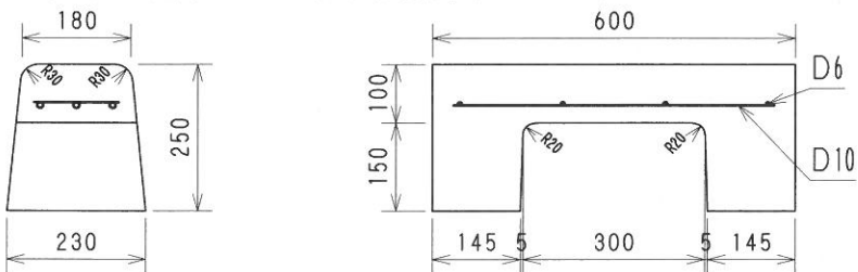
両面歩車道境界ブロック(B)水抜部(O-10型) 180/230×250×600
