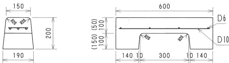
両面歩車道境界ブロック(A)水抜部(O-9型) 150/190×200×600 ※( )内寸法の製品もあります。
