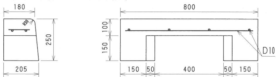
片面歩車道境界ブロック(B)水抜部 180/205×250×800
