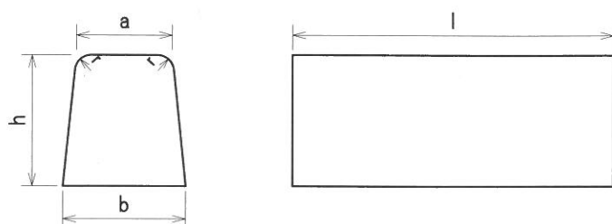
(両面歩車道境界ブロック)
