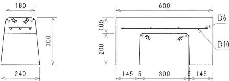
両面歩車道境界ブロック(C)水抜部 180/240×300×600
