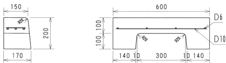
片面歩車道境界ブロック(A)水抜部 150/170×200×600
